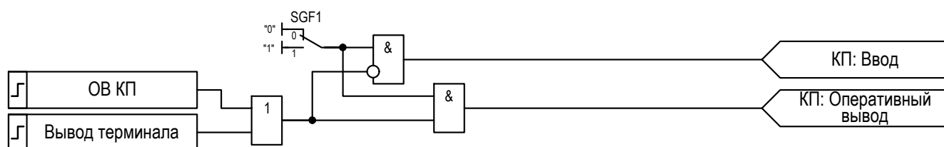
Рисунок 2.8 – Функциональная схема управления режимами работы «КП»
