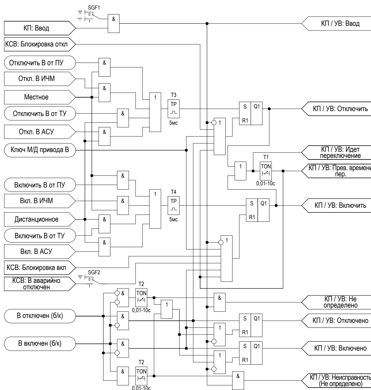
Рисунок 2.9 – Функциональная схема «УВ»
