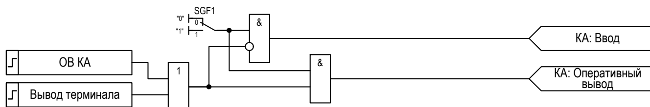
Рисунок 2.10 – Логика управления режимами функционального блока «КА»
